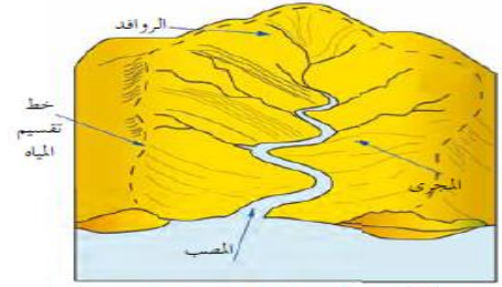
الشكل رقم (٣-٢٨) : حوض نهري.
