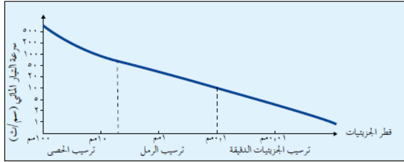
الشكل رقم (٣-٣): العلاقة بين سرعة النهر (سم/ث) وحجم الرواسب.
