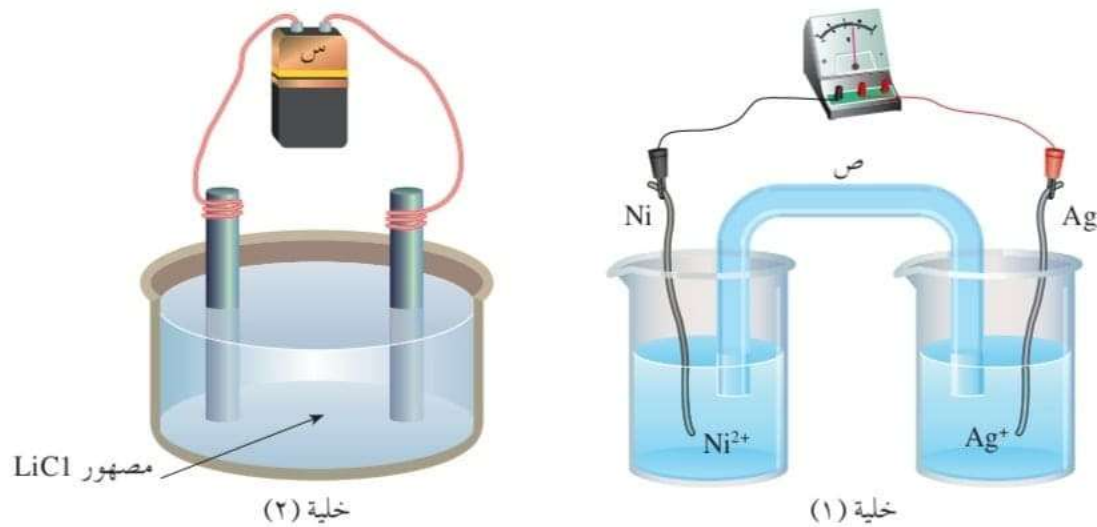
الشكل (٢-١٥): خليتان كهركيميائيتان.
