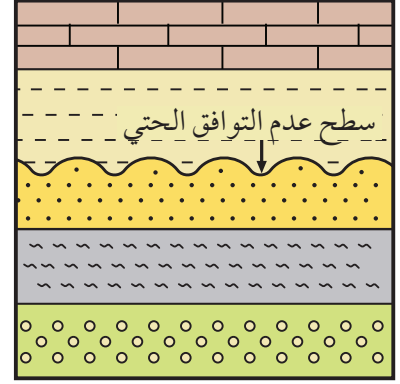
الشكل (17): طبقات متوازية يفصل بينها سطح عدم التوافق الحَتِّي.
