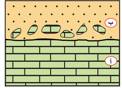
الشكل (15): احتواء الجسم الصخري (ب) قطعاً صخرية من الجسم الصخري (أ).
