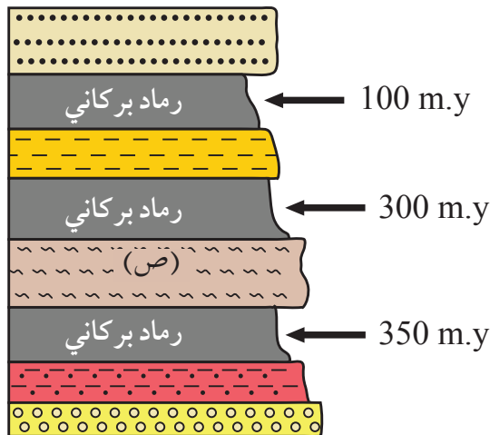
الشكل (24): تُستخدَم طبقات الرماد البركاني في تحديد عُمر الصخور الرسوبية. أستخدم عُمر الطبقة الرسوبية (ص)؟
