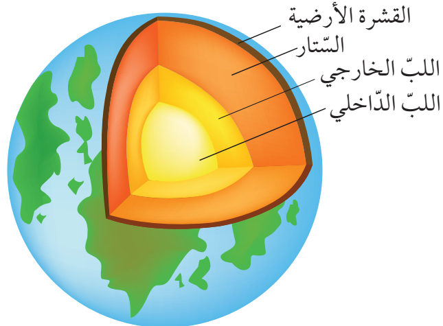
الشكل (4) أنطقة الأرض الرئيسة كما تمايزت بعد تشكّل الأرض.
