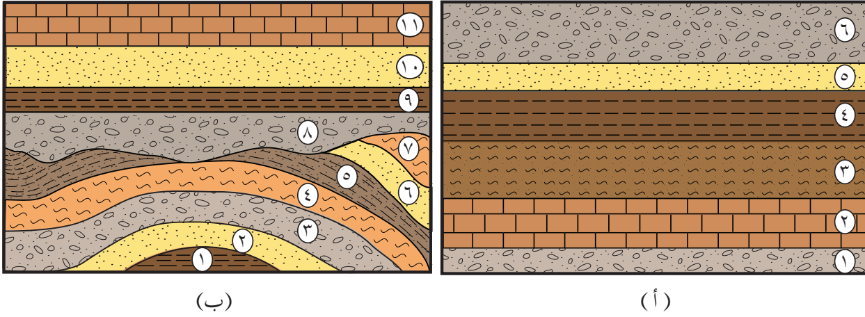
الشكل (٣-١٧): مبدأ الترسيب الأفقي ومبدأ تعاقب الطبقات.
