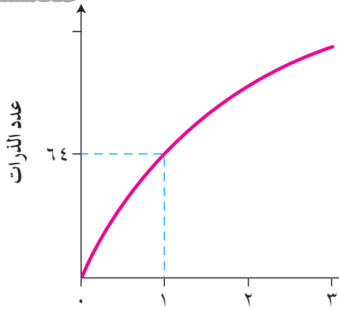
عدد فترات عمر النصف (ن) الشكل (٣-٣٣): السؤال (٤).
