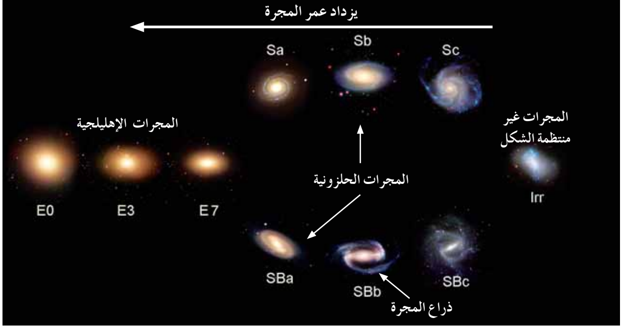
الشكل (١٤-١): مخطط الشوكة الرّنانة لتصنيف المجرات.
