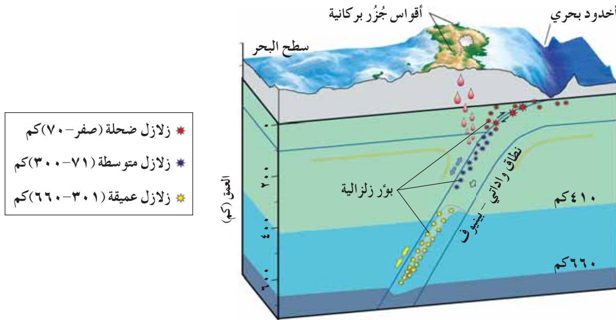
الشكل (٥-٢٨): توزع البؤر الزلزالية عند نطاق الغوص (نطاق وادائي - بينيوف).
