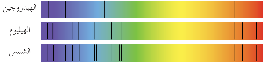
الشكل (١-٦): طيف امتصاص الهيدروجين والهيليوم في طيف الشمس. وقد تم التركيز على طيفي امتصاص الهيدروجين والهيليوم؛ لأنهما يشكلان المكوّنات الرئيسة للشمس ونسبة ٩٨٪ تقريباً.
