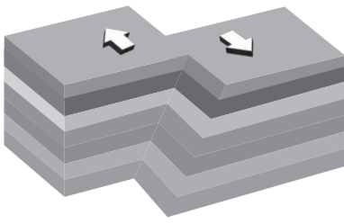
صدع جانبيّ
