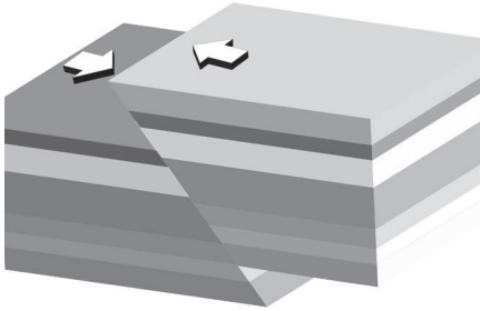
الصّدع العكسيّ
