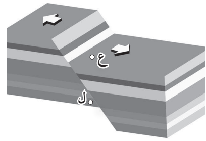
صدع عاديّ
