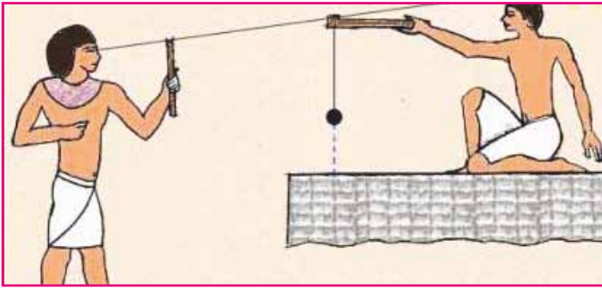
الشكل (١-١٤): حساب الزوايا عند المصريين القدماء.
