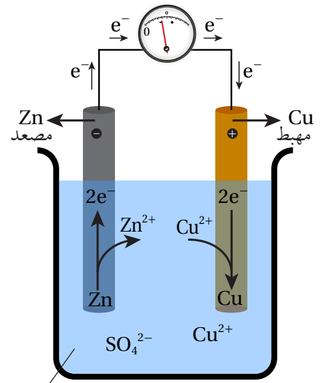
\text{CuSO}_4(\text{aq})
